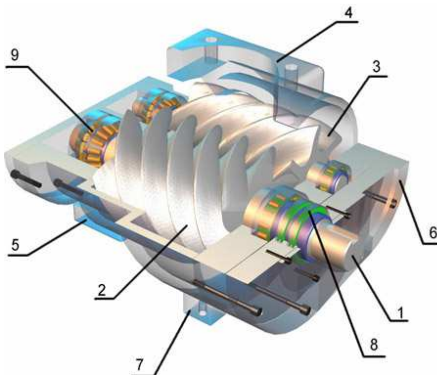
Винтовой блок.
